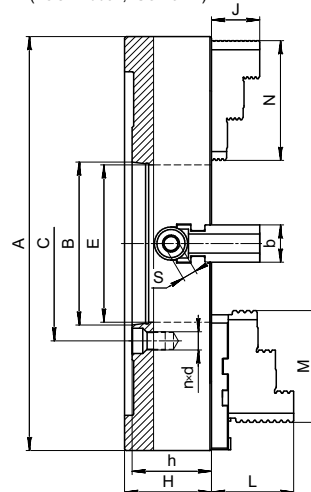
Тип крепления 4 «D» (ГОСТ 26651; ISO 702-2)
