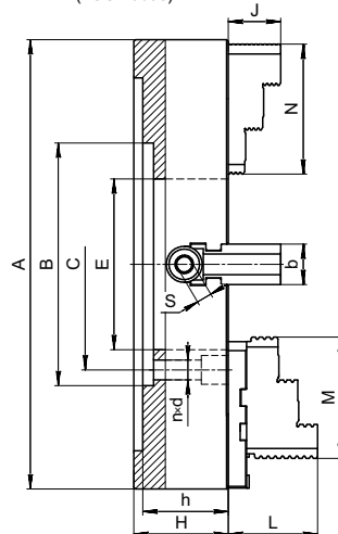
Тип крепления 3 «C» (ГОСТ 3890)
