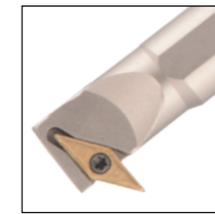
SVZ□□93°
