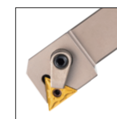
MTGN□91°
