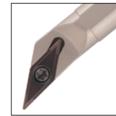
SVX□□96°
