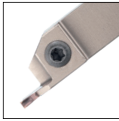
KGM□
