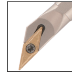
SVJ□□93°
