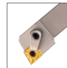
MCGN□91°
