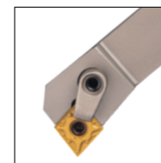
MCFN□91°
