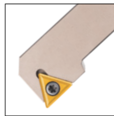
STGC□91°
