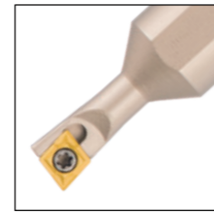
SCLC□-A 95°
