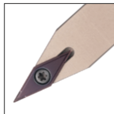
SVVC/BN72.5°
