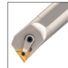
MTUN□95°
