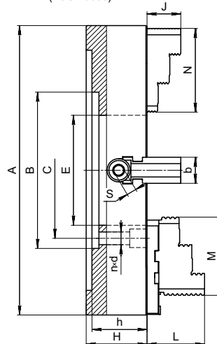
Тип крепления 3 «C» (ГОСТ 3890)
