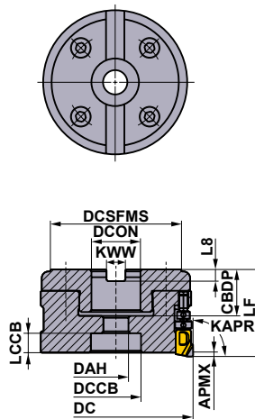
Рис.2 ø3.000" ø4.000" ø80mm
